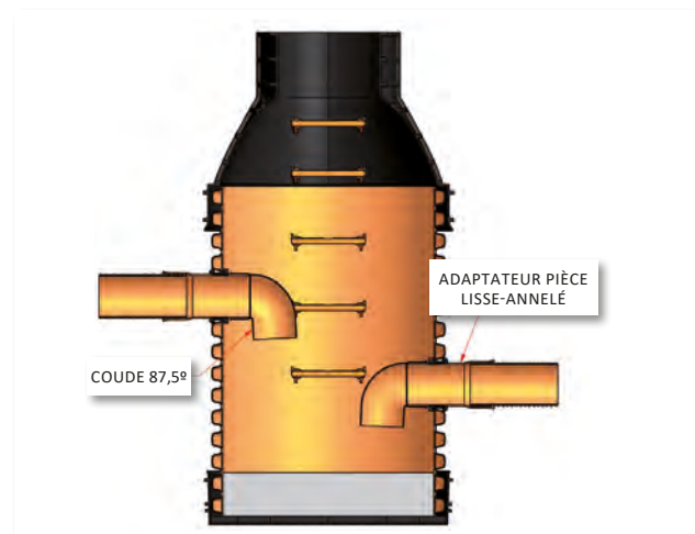
REGARDS SÉPARATEURS DE GRAISSES
