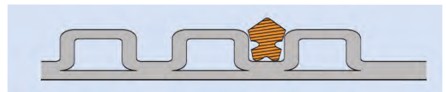
JOINT À ANCRAGE SIMPLE SUR SANECOR® DN630-1200
