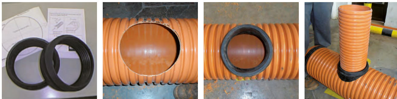
CLIPS EN ÉLASTOMÈRE AVEC GABARIT DE COUPE POUR BRANCHEMENTS
