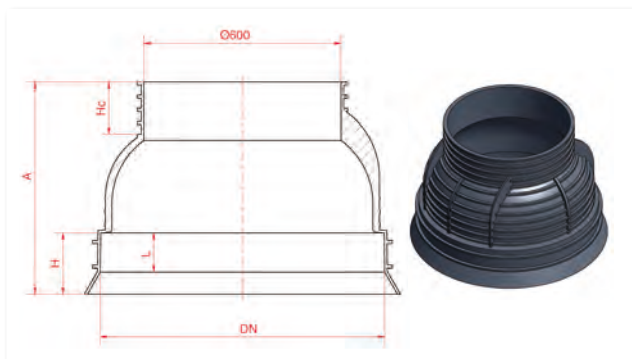
CÔNE RÉDUCTEUR DE REGARD DE DIAMÈTRE 800 MM
