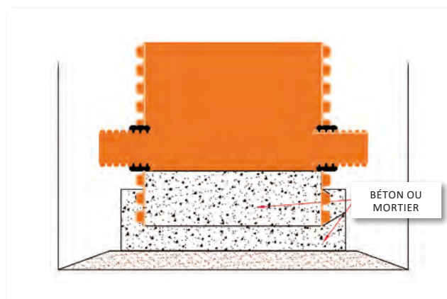
FINITION DU REGARD AVEC BÉTON 2ÈME PHASE
