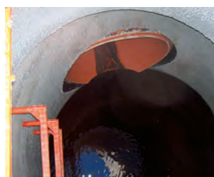
MANQUE D'ÉTANCHÉITÉ SUR REGARDS EN BÉTON
