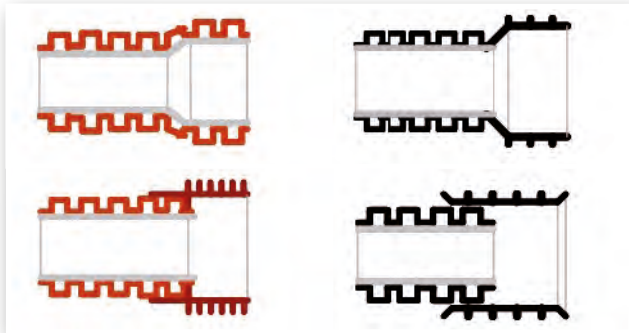
DIFFÉRENTS SYSTÈMES D'UNION DE TUYAUTERIES EN PLASTIQUE STRUCTURÉES
