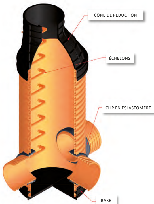
SCHEMA GÉNÉRAL DE REGARDS SANECOR®
