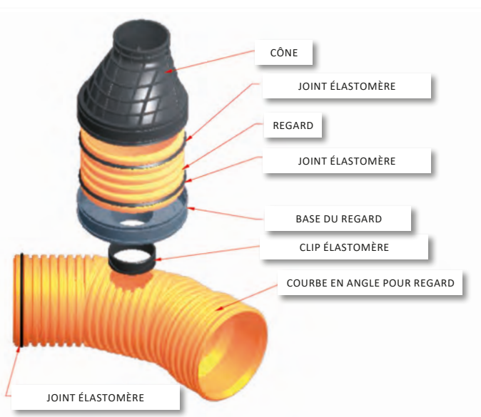
INSTALLATION DE REGARDS SUR COLLECTEURS AVEC CHANGEMENT DE DIRECTION
