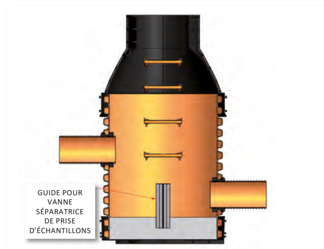
REGARDS POUR PRISE D'ÉCHANTILLON
