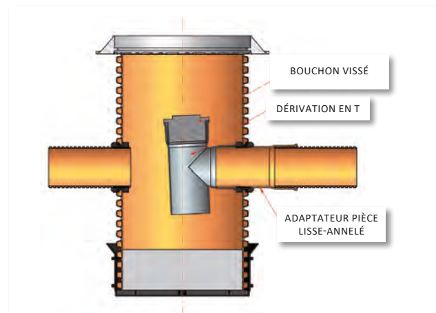
REGARD SIPHONIQUE
