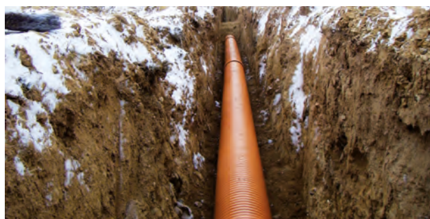
VUE DE TUBE SANECOR® INSTALLÉE DANS LE FOSSÉ
