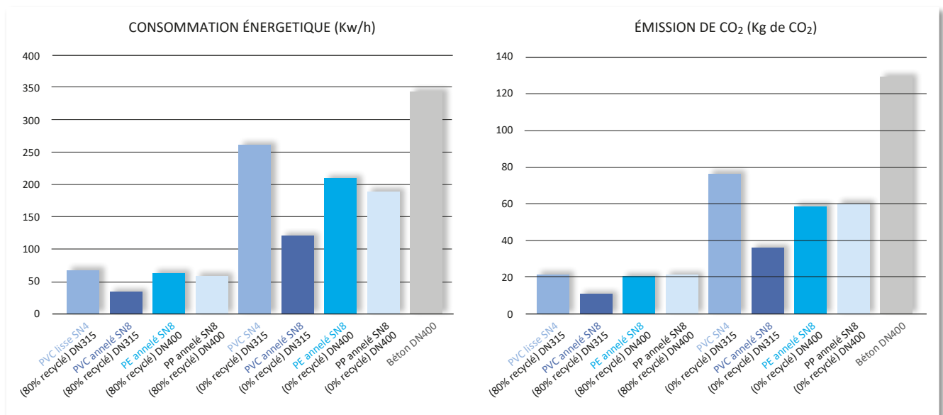
GRAPHIQUES DE LA CONSOMMATION ÉNERGETIQUE ET D'ÉMISSION DE CO 2 DANS L'ATMOSPHÈRE DES MATÉRIAUX LES PLUS UTILISÉS SUR LES TUYAUTERIES D'ASSAINISSEMENT PAR GRAVITÉ
