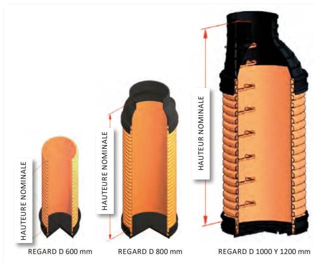
GAMME STANDARD DE CORPS SANECOR®
