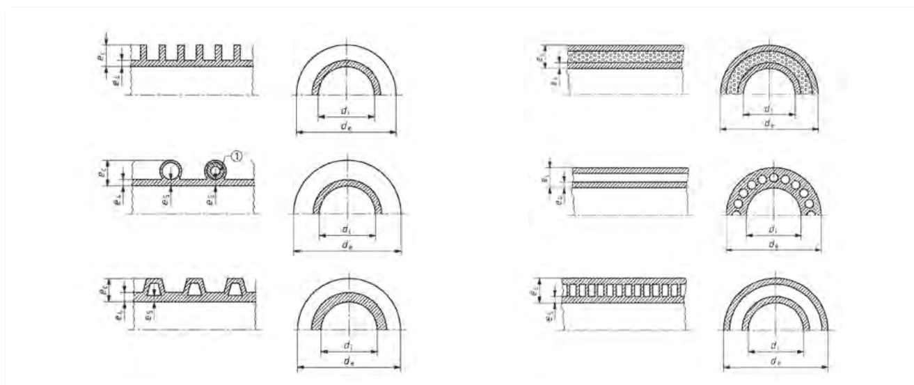
PRINCIPAUX PROFILS UTILISÉS SUR TUYAUTERIES STRUCTURÉES
