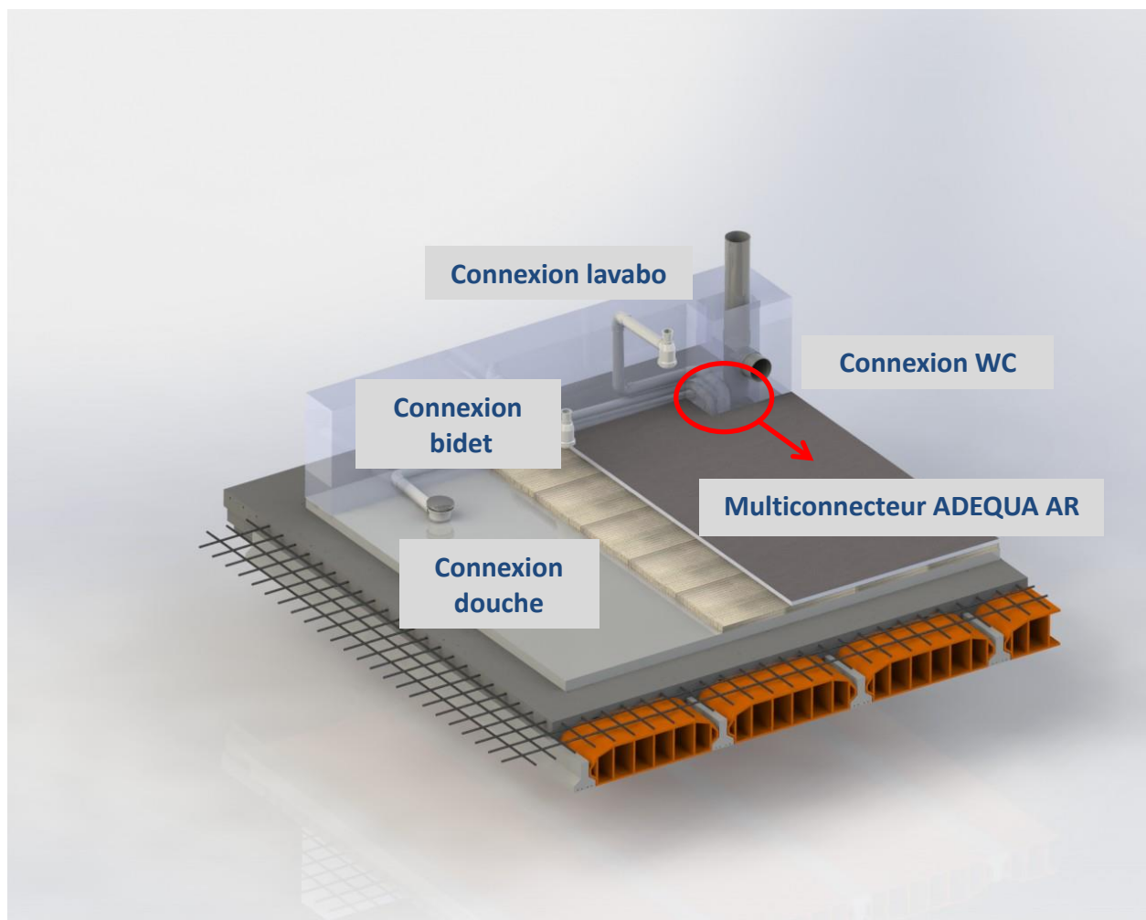
Figure 4 - Schéma d'installation du Multicconnecteur ADEQUA AR : connexion d'une salle de bain
