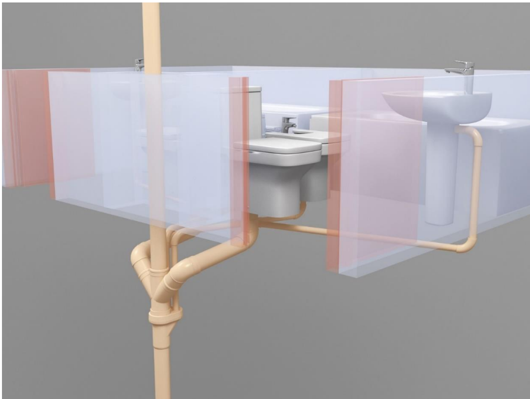
Figure 5 - Schéma d'installation du Multiconnecteur ADEQUA AR : connexion de 2 salles de bains symétriques
